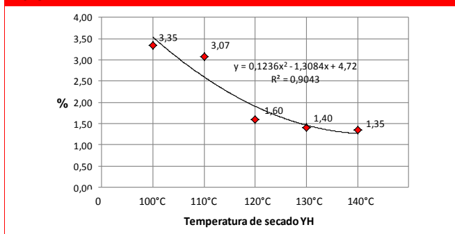
Figura 3. Agua combinada en residuos YH. Fuente: Elaboración Propia, 2013.
