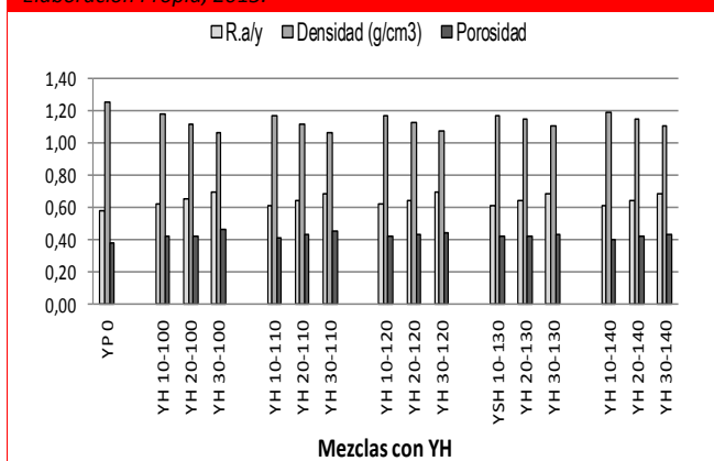
Figura 7. Relaciones a/y-Densidad-Porosidad. Mezclas con YH. Fuente: Elaboración Propia, 2013.
