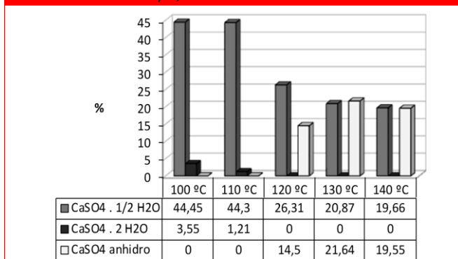
Figura 4. Contenido de los diferentes sulfatos de calcio en residuos YS. Fuente: Elaboración Propia, 2013.
