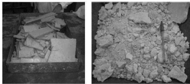
Figura 1. Izq.: Yeso recuperado de placas (YS). Der.: Yeso recuperado de aplicaciones húmedas (YH). Fuente: Elaboración Propia, 2013.
