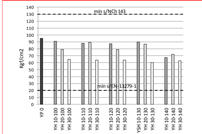
Figura 11. Prismas (YH). Resistencia a la compresión. Fuente: Elaboración Propia, 2013.
