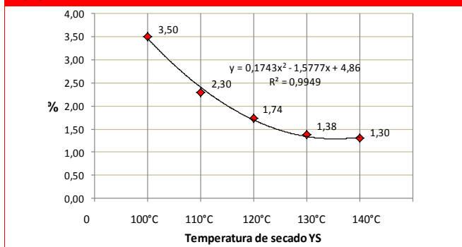
Figura 2. Agua combinada en residuos YS. Fuente: Elaboración Propia, 2013.
