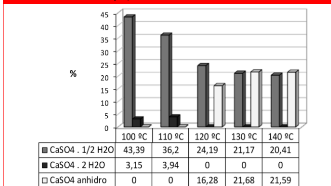
Figura 5. Contenido de los diferentes sulfatos de calcio en residuos YH. Fuente: Elaboración Propia, 2013.
