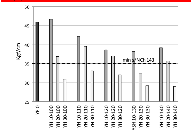
Figura 9. Prismas (YH). Resistencia a la flexión. Fuente: Elaboración Propia, 2013.
